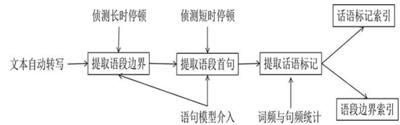
图3 话语标记自动提取流程
